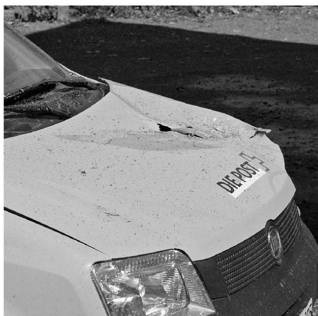
Fig. 9: Schlagspuren durch Steinschlag an PW vor der Talstation.
