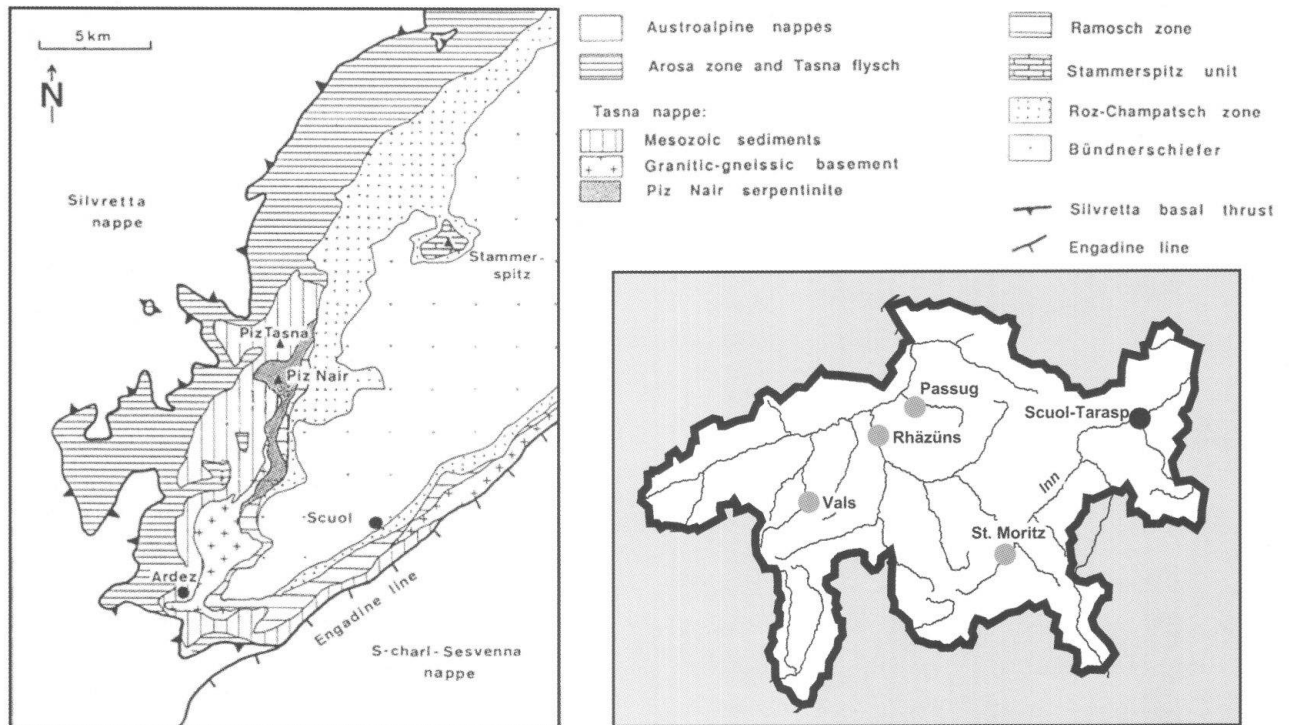
Fig. 1: Links: Tektonische Übersicht des Unterengadins in der Gegend von Scuol (aus Florineth & Froitheim 1994). Rechts: Geografische Übersichtskarte des Kantons Graubünden.
