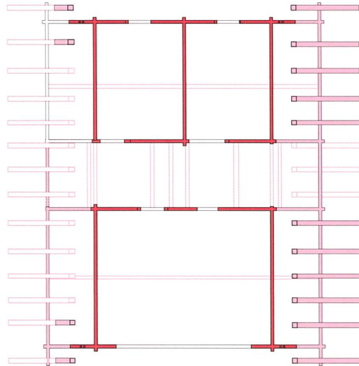
Grundriss Dachgeschoss
