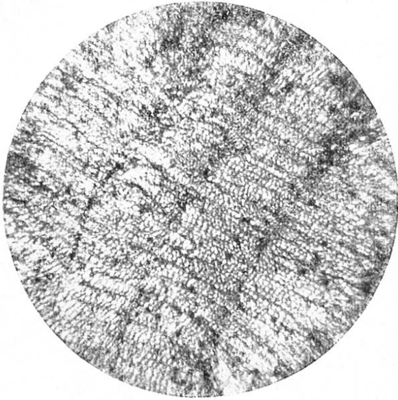
Radialer Querschnitt. 20 : 1.
