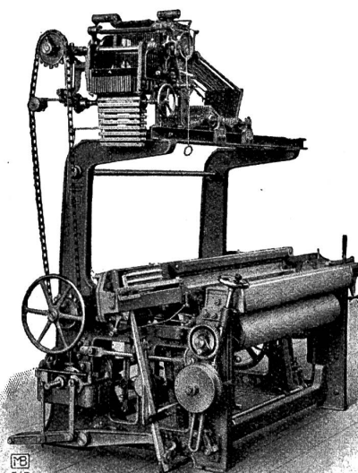
Vierschützig einseitiger Wechselstuhl
