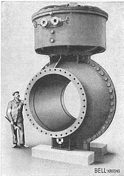
Bell-Kugelschieber von 1400 mm Durchmesser, nach Spanien geliefert
