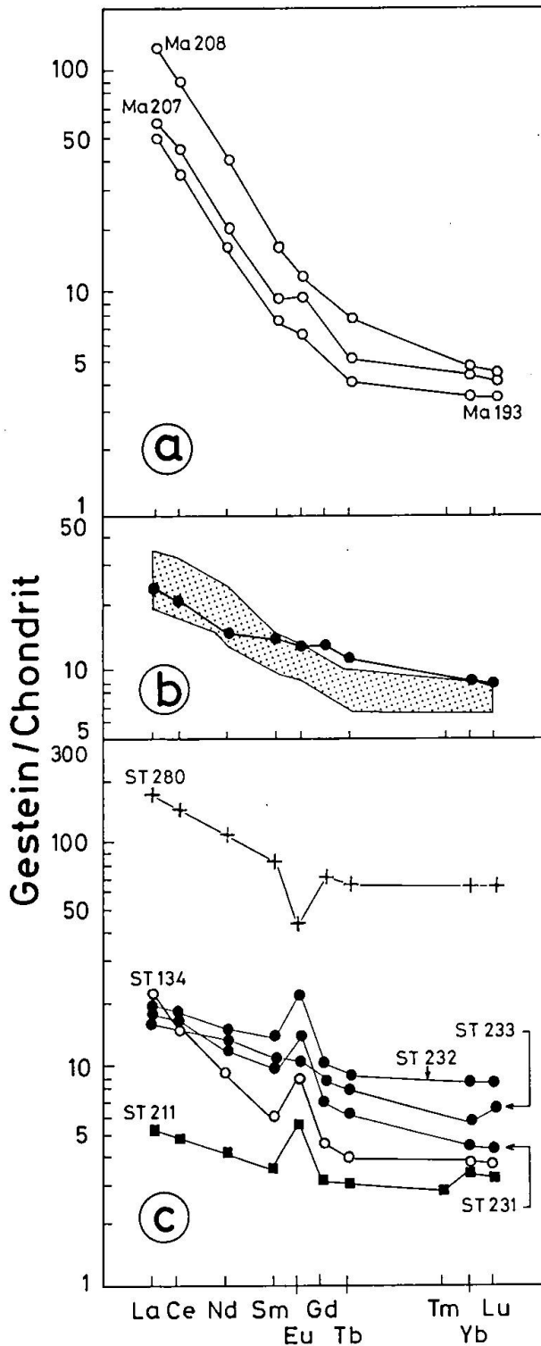
Abb. 3 Chondrit-normierte SE-Verteilungsmuster diverser «Älterer Orthogneisse».
