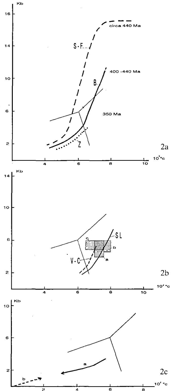
Fig. 2 Evolution tectono-métamorphique
