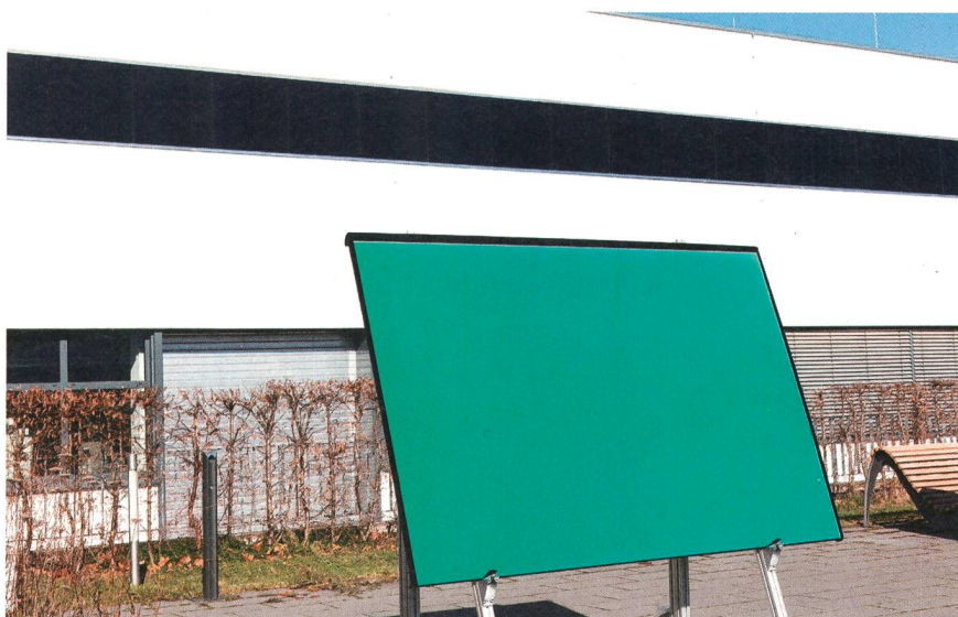
Die grünen PV-Module liefern 195 W - 93% der Leistung der schwarzen auf der Fassade.
