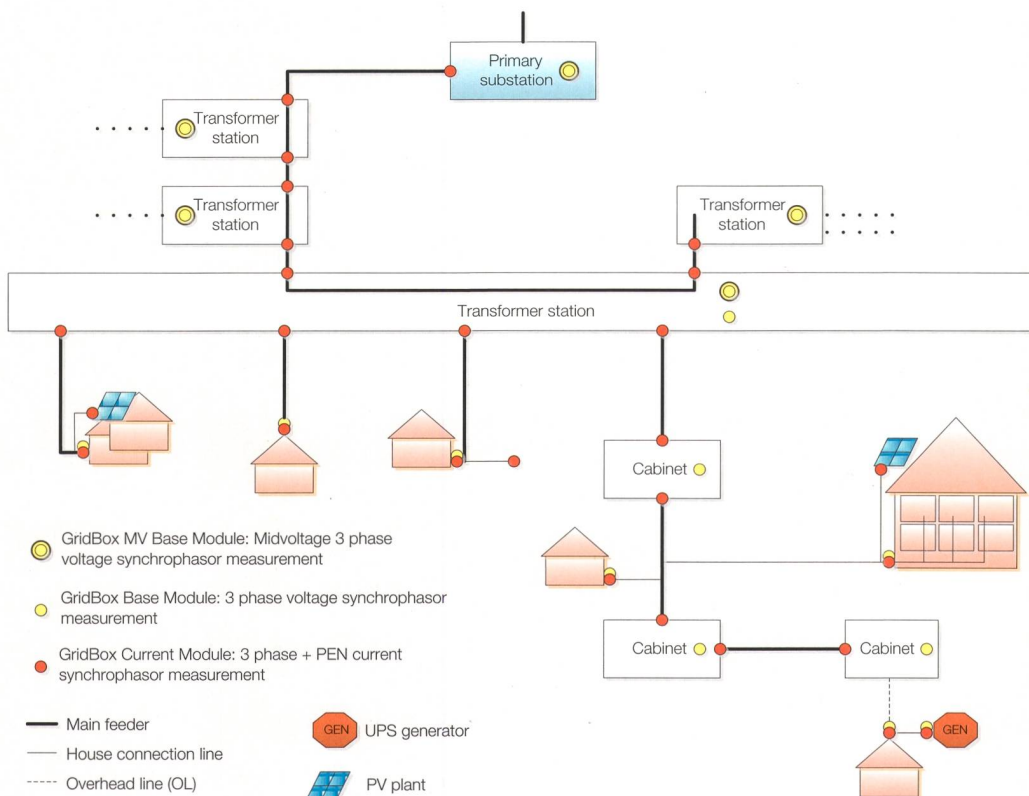
Bild 1 Schematisches Gridbox-Pilotnetz.
