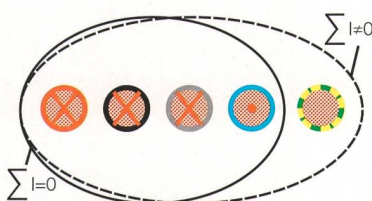
Bild 1 Typisches Drehstromsystem.
