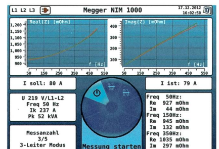
NIM 1000 protokolliert die Impedanz bis zur 10. Harmonischen.
