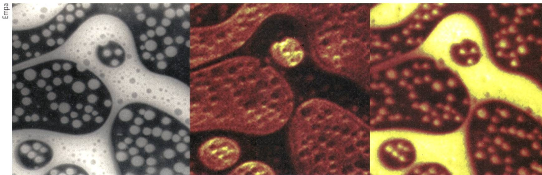
Le SFM reproduit topographiquement la surface de l'échantillon (12µm x 12µm, à gauche) alors que le TOF-SIMS met en évidence la localisation des polymères qui la constituent (au centre, les ions C - et C 2- et à droite, les ions CN - et I + ).
