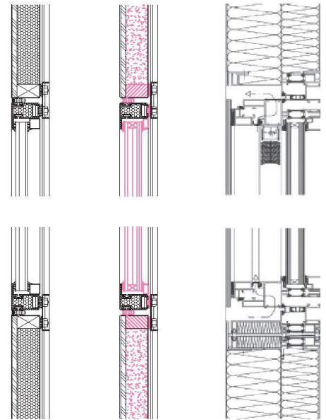
02 Vertikalschnitte durch Fassade und Verglasung. Von links nach rechts: Bestand, Vorschlag Komitee, Vorschlag AGG (Mst. 1:10) (Pläne: Komitee «Rettet den Gymer Strandbode!» / AGG)
