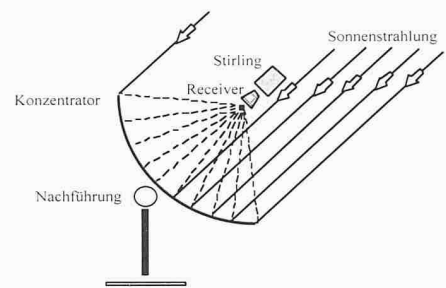
3 Schematische Darstellung eines Dish/Stirling-Systems [5] (Bild: Schlaich Bergemann und Partner)
