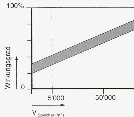
3 Speicherwirkungsgrad in Funktion des Speichervolumens V_s (Höhe/Durchmesser = 1, Dicke der Wärmedämmung an der Speicher- oberseite: 0,3 m)
