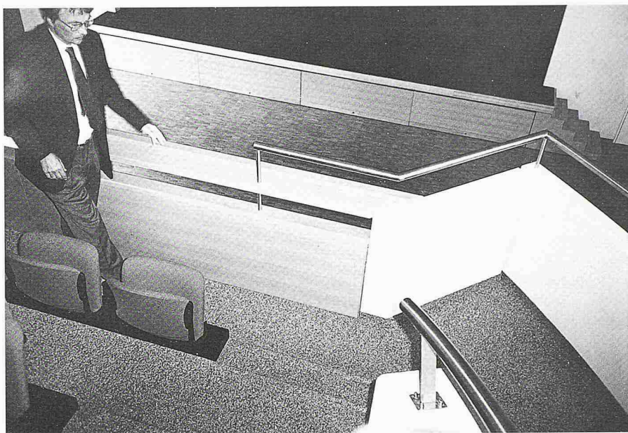
Fusspunkt der Erschliessungstreppe für die oberen Tribünenreihen mit einem normkonformen Geländer von 100 cm Höhe
