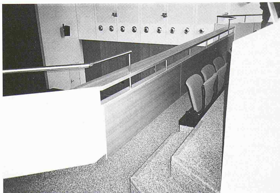
Auf 25 cm verbreiterte Krone der Brüstung von 80 cm Höhe bei der vordersten Sitzreihe der Tribüne
