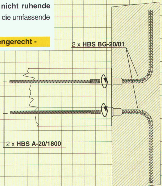
Grundriss-Detail
