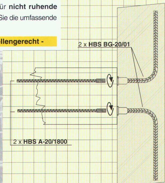
Grundriss-Detail
