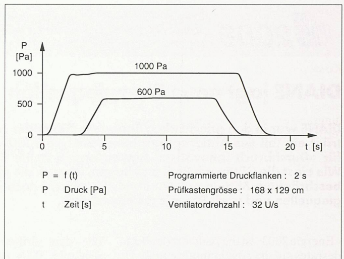
Bild 3. Druckpulse
