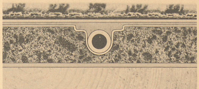
Mit nur 25 mm Aufbauhöhe eignet sich die Fussbodenheizung Stramax R25 für den gesamten Sanierungsbereich
