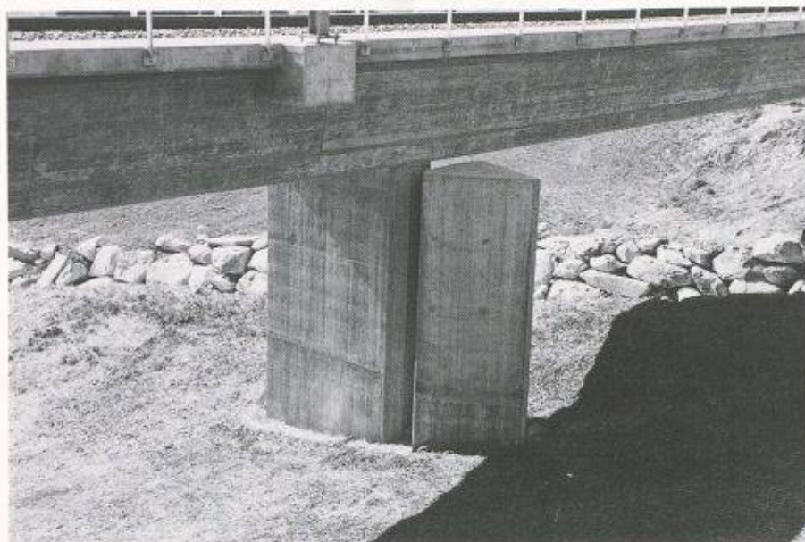
Bild 5. Lawinenspaltkeil
