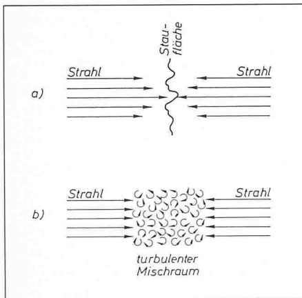
Bild 16. Schema des Staustrahlreaktors
