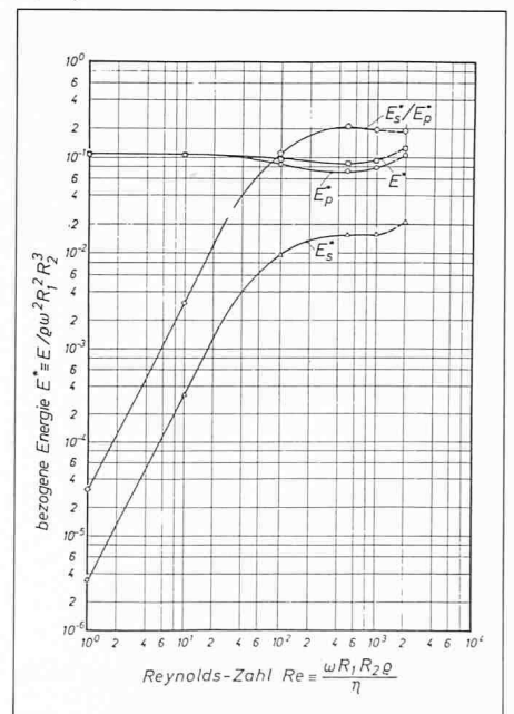
Bild 12. Energien in der Primärströmung E_p^* und in der Sekundärströmung E_s^* sowie das Verhältnis E_s^*/E_p^* in Funktion der Reynolds-Zahl Re_{12}
