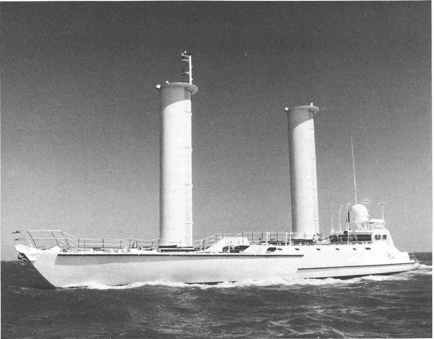
Bild 5. Turbosegelschiff «Alcyone»
