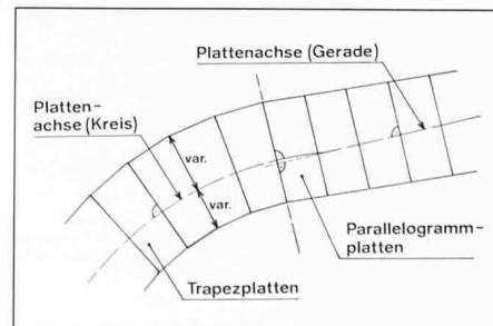
Bild 2. Grundrisseinteilung der Platten
