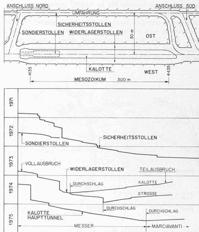
Bild 7. Ablauf der Bauarbeiten im Bereich des «Mesozoikums»
