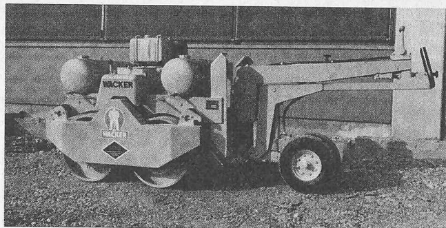
Wacker-Doppelvibrwalze Typ W 85 L mit Lenkschemel Generalvertretung für die Schweiz: MBA, 8600 Dübendorf Tel. 01/85 00 21
