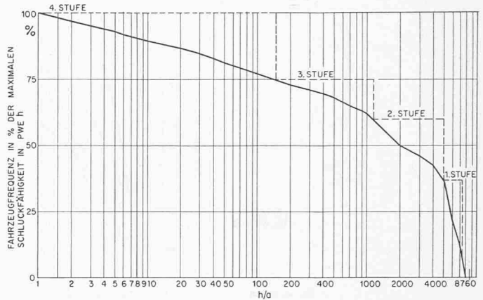
Bild 2. Verkehrsdauercurve
