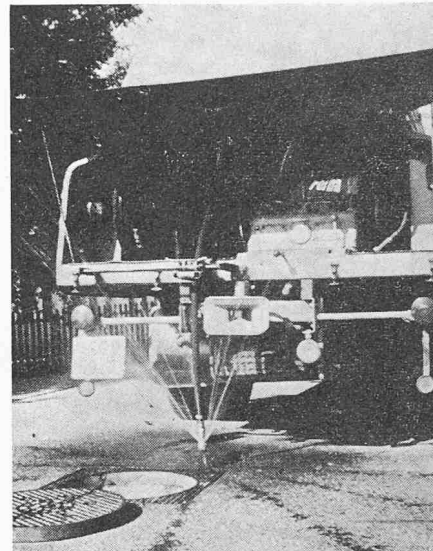
Bild 9. Kanal-Hochdruckreinigungsgärat
