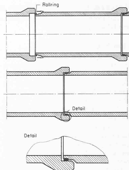
Bild 3. Schematische Darstellung des Abdichtens von Glockenmuffen mit Rollringdichtung
