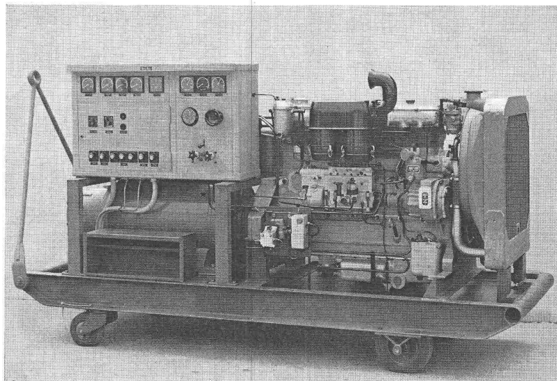
Fahrbare Notstromgruppe für 60 KVA Leistung, 6-Zylinder-Saurer-Dieselmotor, Dauerleistung 80—90 PS bei n = 1500 t/min.
