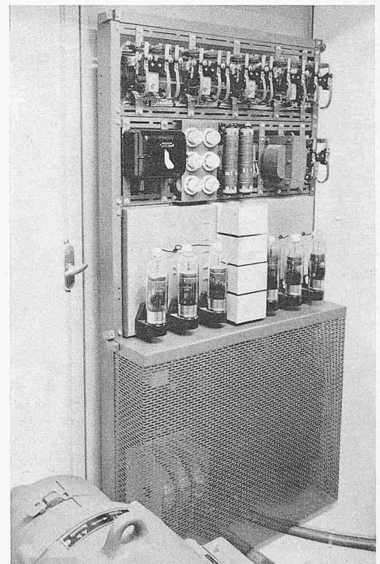
Bild 3. Geöffneter Apparateschrank eines Monotronaufzuges. Oben Schütten zum Ein- und Ausschalten, für Fahrtrichtungswechsel sowie Schaltung der verschiedenen Fahrphasen. Auf mittlerer Höhe in der Mitte Thyatron zur Regulierung des Motors. Unten das zur Steuerung der Thyatron nötige Verstärkergerät, das Drehknöpfe zum Einregulieren der Laufeigenschaften (Beschleunigung, Verzögerung usw.) enthält.
