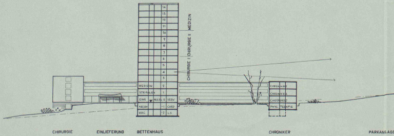
Querschnitt Bettenhaus, M. 1:1000
