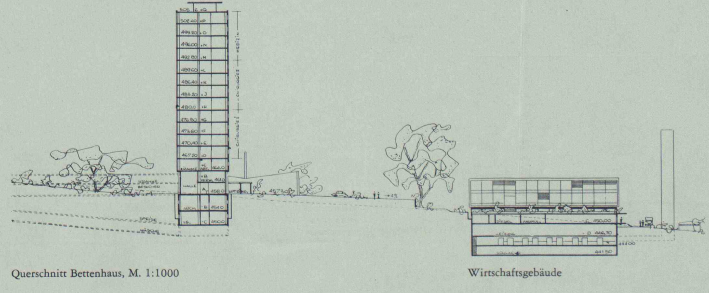
Querschnitt Bettenhaus, M. 1:1000
