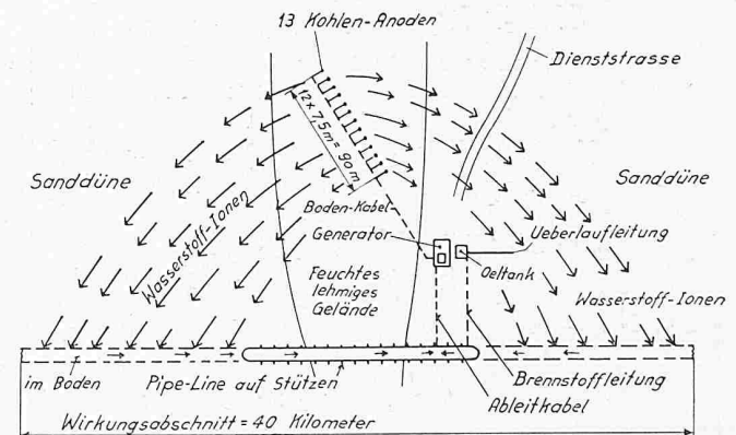
Bild 7. Installationsschema einer «Cathodic Protection»-Anlage. Die 13 Anoden sind auf eine Länge von etwa 100 m in Abständen von je 7,5 m eingegraben
