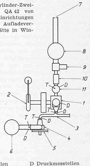
Bild 5 (rechts). Einrichtungen zur Untersuchung des Stossverfahrens am aufgeladenen Zweitakt-Dieselmotor 1 QA 42
