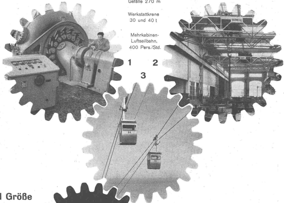
Francisturbine von 22 350 PS, Gefälle 270 m
