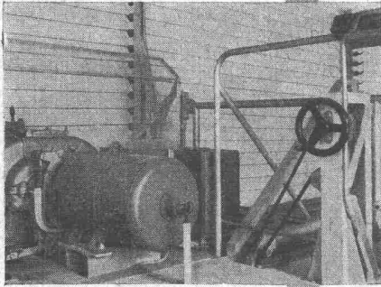
Elektronisch gesteuerte Flügelprüfanlage für stufenlosen Regelbereich von 1:900
