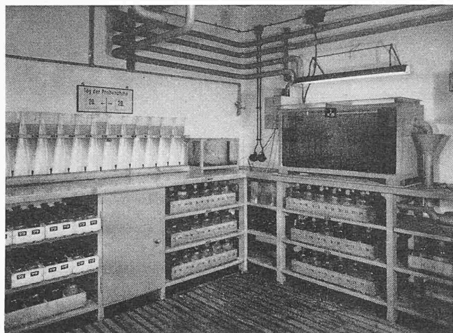
Bild 22. Blick in die Kontrollstation mit den Probenahmegefäßen
