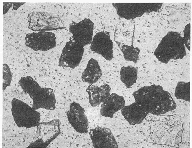
Bild 4. Mikroskopisches Präparat der Siebfraktion 0,06 — 0,09 mm eines PCS5, wie sie zum Auszählen des Schlackengehaltes verwendet werden. Farblose Körner mit «glasigem» Bruch = Hochofenschlacke; die übrigen dunklen Körner = PC-Komponenten. Durchfallendes Licht; Vergrösserung rd. 150fach
