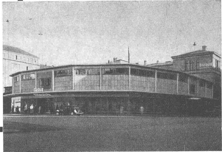
Ausfachung eines Stahl-Skelettbaues
