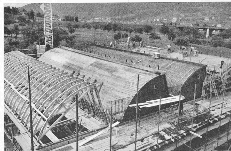
Bild 7. Schalen und Armieren. Links sind die Lehren sichtbar, auf welche die Schalungstafeln verlegt werden. (Textilwerk Hanro in Liestal, Ausführung Preiswerk & Co., Basel)
