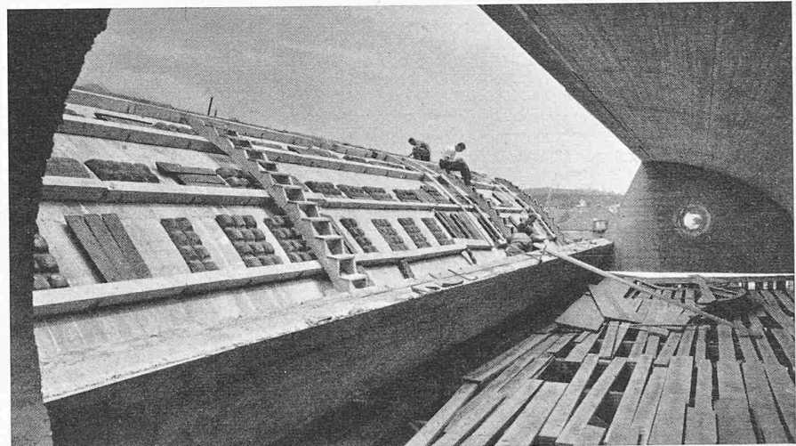
Bild 6. Probelastung von Shed Nr. 2 mit einer verteilten Last von total 24 t
