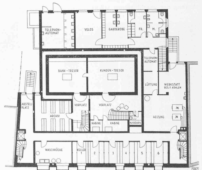
Bild 14. Keller 1:350
