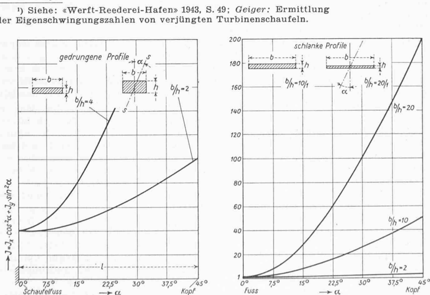
Bilder 1 und 2. Abhängigkeit des Trägheitsmomentes eines Rechteckquerschnitts, wenn die Schwingungsrichtung S-S von der Trägheitshauptaxe um den Winkel \alpha abweicht
