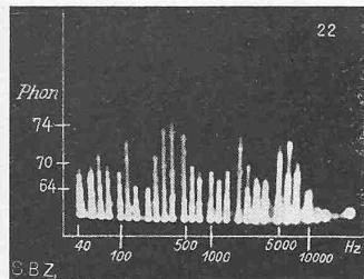
Tonfrequenz-Spektre : Abb. 7. Geräusch in Bahnhofhalle
