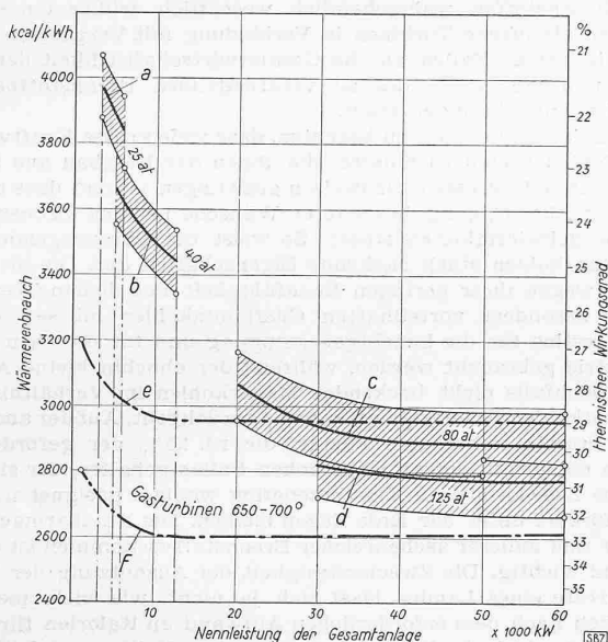
Abb. 5. Ungefähre spezifischer Wärmeverbrauch und thermischer Wirkungsgrad von Gas- und Dampfturbinen in Abhängigkeit der Nennleistung bei Verfeuern von Steinkohle und bezogen auf die nutzbar abgegebene Leistung
