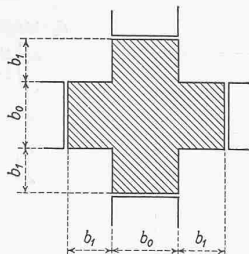
Abb. 7. Fugen im Schwellenrost
