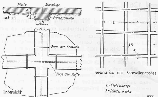
Abb. 5. Betonplatte mit Randschwellen
