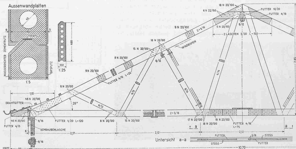
Abb. 11. Dachbinder in Holz-Nagelbau, 1:50
