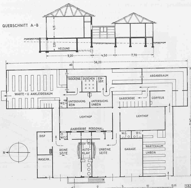
Abb. 1. Grenz-Notspital Schaffhausen Grundriss 1:400 der Desinfektionsanlage
