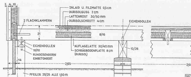
Abb. 9. Boden- und Wandkonstruktion 1:30
