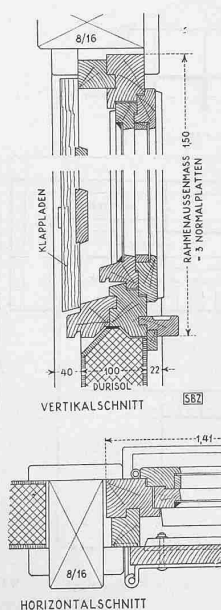
Abb. 10. Fensterdetail 1:10; Plattendetail 1:5 und 1:25
