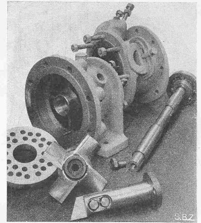
Abb. 2. Bestandteile der Pumpe Abb. 1
