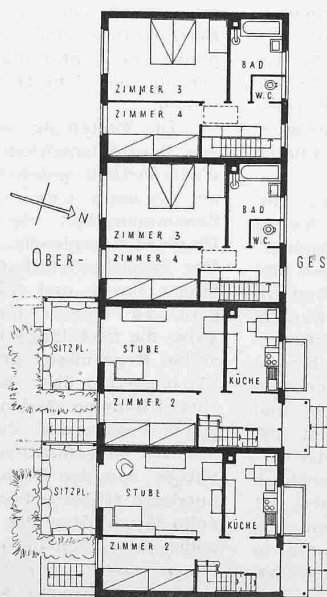
OBER- ERDGESCHOSS Masstab 1:300
