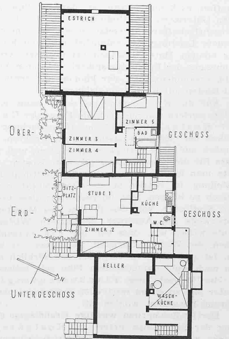
OBER- ERD- UNTERGESCHOSS Fünfzimmer-Einfamilienhäuser, südlicher Block A
