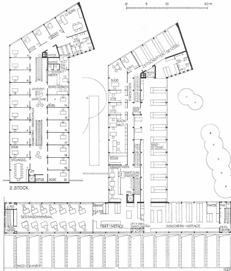
Abb. 10. Obergeschosse. — Masstab 1 : 500
