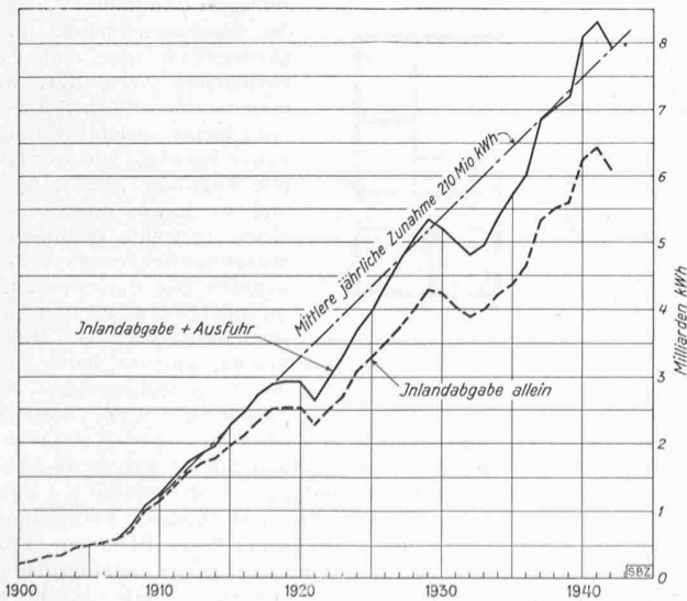
Abb. 23. Entwicklung der Energieabgabe der Schweiz, Elektr.-Werke
