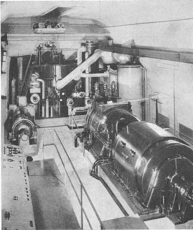
Abb. 6. Bombensichere Zentrale Bern von 5000 kW Leistung. Ein Veloxkessel, im gleichen Raum mit der Dampfturbine aufgestellt, erlaubt die Vollleistung innerhalb 10 min vom kalten Zustand aus zu erreichen
